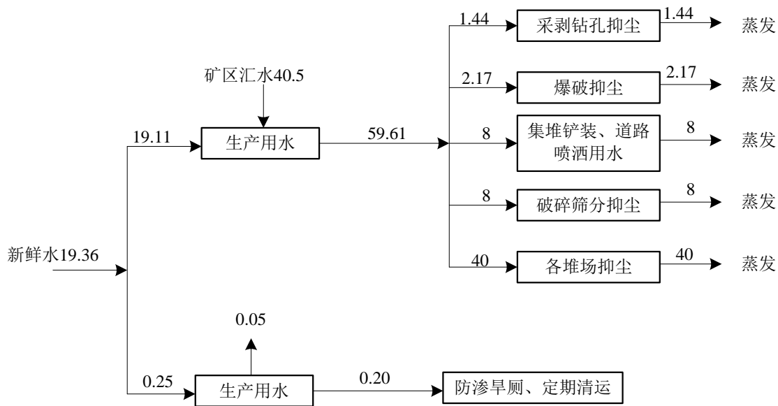
图 3-2-2 水平衡图 单位 (t/d)
